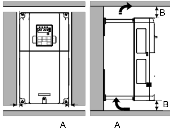
Рисунок 4-2. Вентиляционные промежутки
