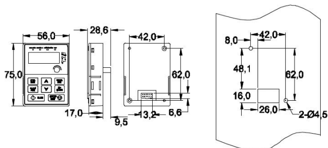
Рисунок 4-4. Настенное крепление
