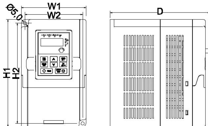
Рисунок 4-3. Габариты преобразователей частоты GD10.
